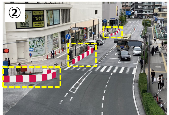
法定で駐停車禁止となっている交差点付近での駐停車対策を行います。ゼブラゾーンや仮設防護柵により、駐停車禁止ゾーンを明確にします。
