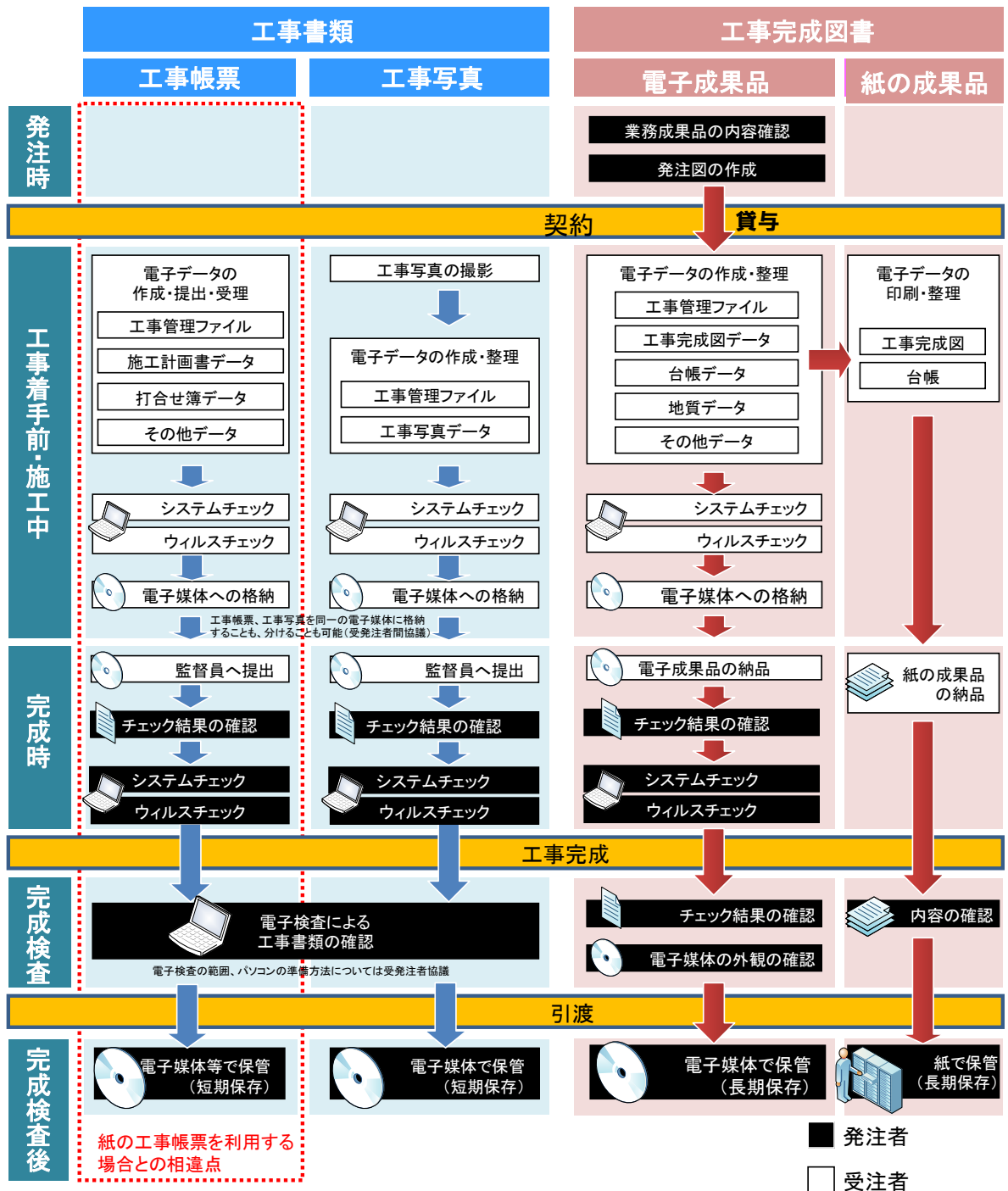
図 2-3 土木工事における電子納品・検査の流れ
