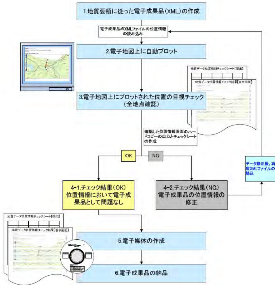
図 6-24 電子地図プロットによる位置情報のチェック全体フロー
