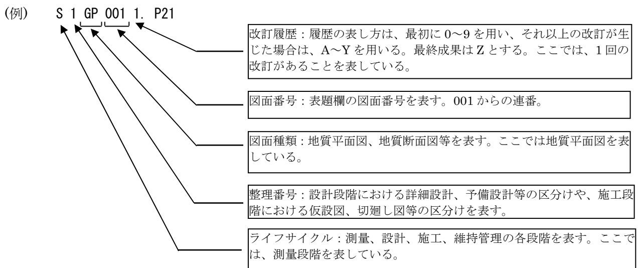
図 6-10 図面のファイル命名
