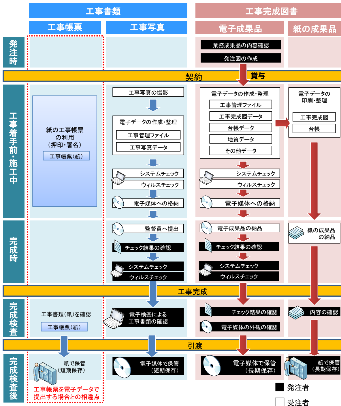
図 2-2 土木工事における電子納品・検査の流れ
