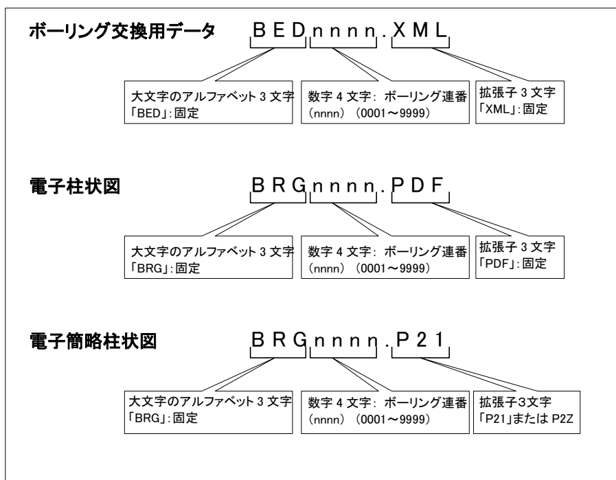
図 6-7 ボーリング柱状図のファイル命名
