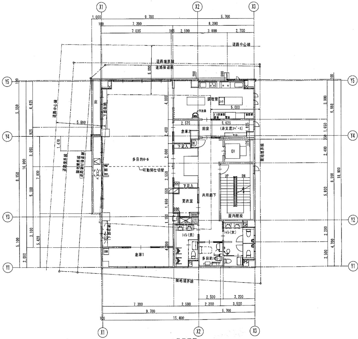
2 階平面図
