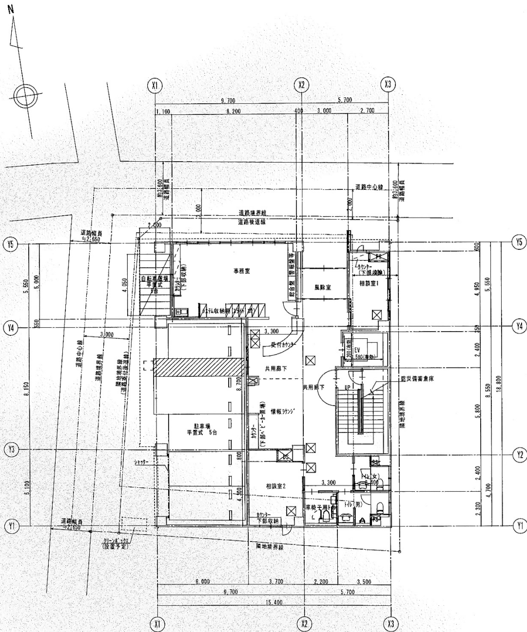
1階平面図
