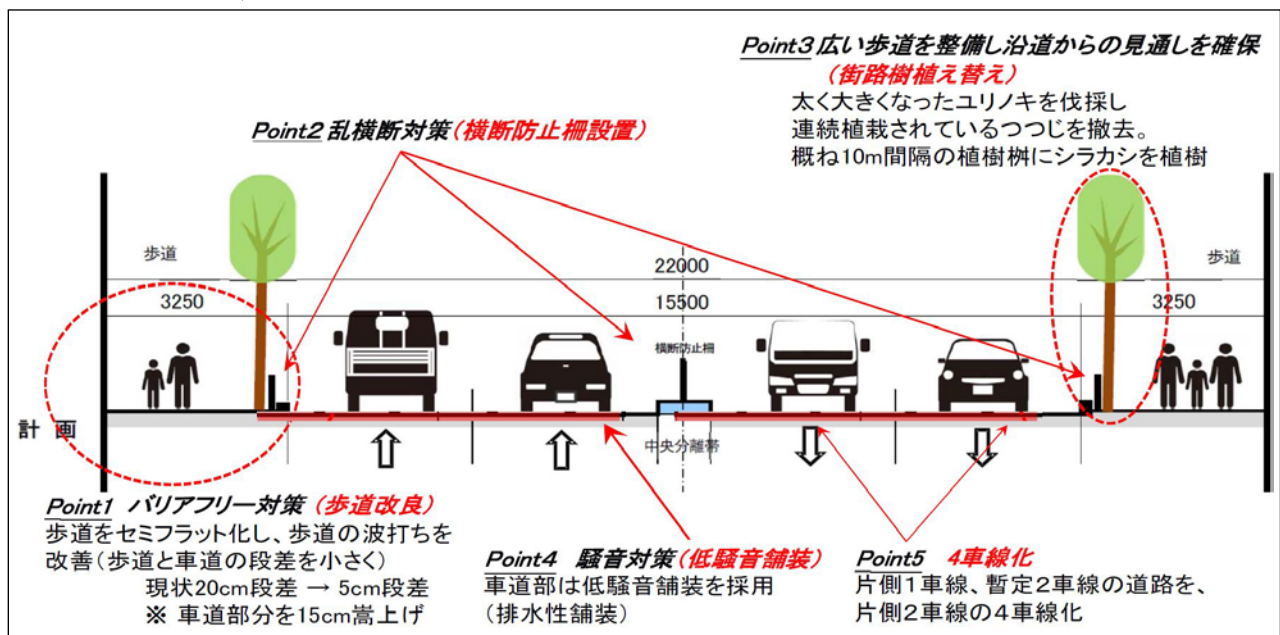
図2 4車線化工事の主な内容
