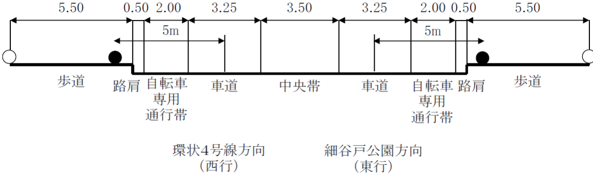
図 6.9-8(5) 道路断面 (地点 5)
