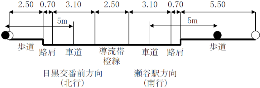
図 6.9-8(6) 道路断面 (地点 6)
