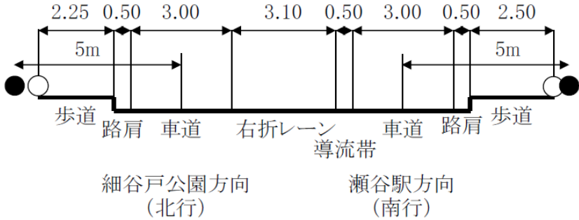
図 6.9-8(7) 道路断面 (地点 7)
