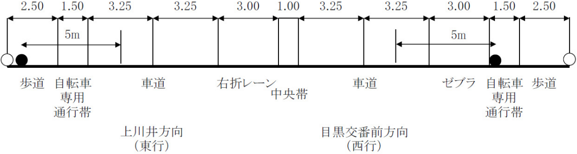
図 6.9-8(3) 道路断面 (地点 3)
