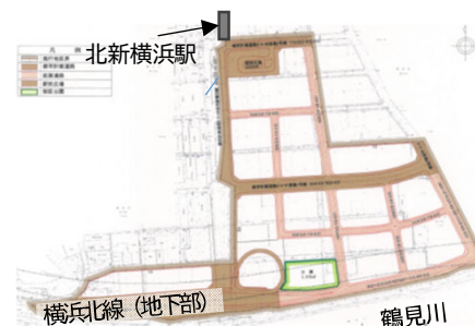
【整備計画図】
