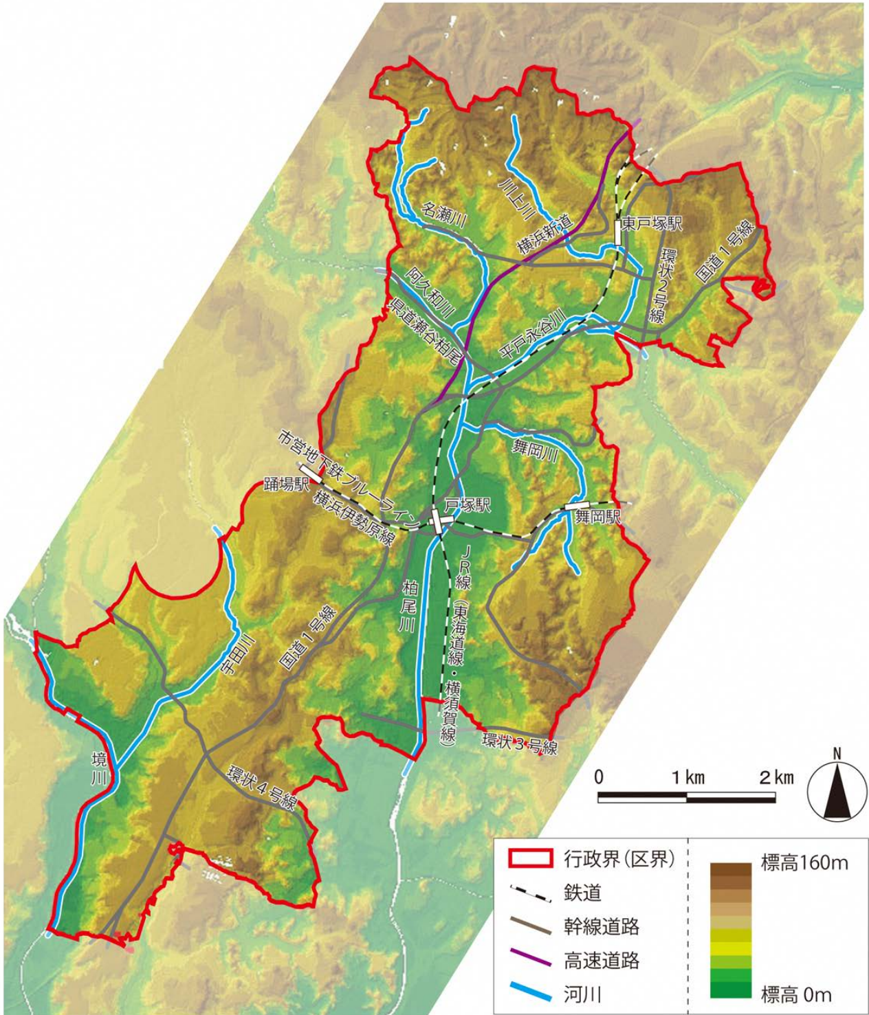
図6 立体地形図
